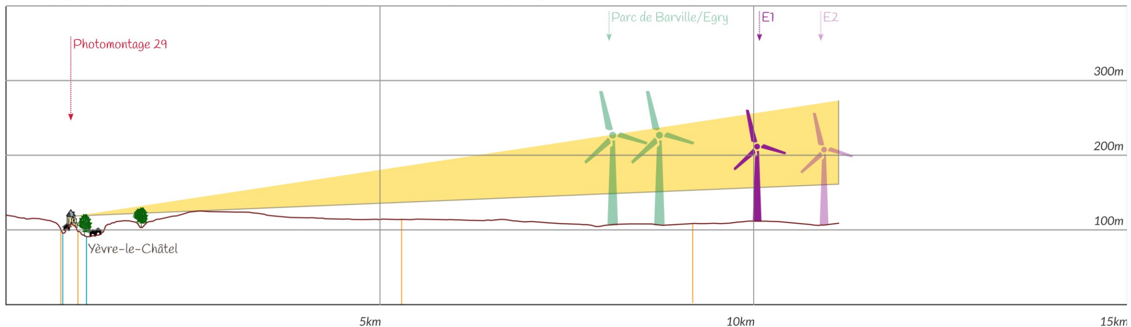
Coupe topographique (Profil Tool d'après IGN BD ALTI 25, Occupation du sol d'après Géoportail, DREAL/DRAC CVdL&IdF)
